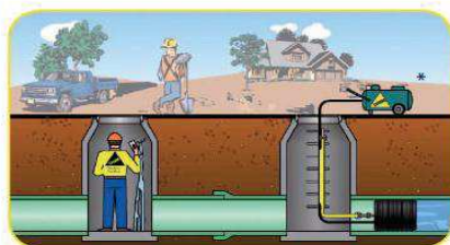
Obturador simple
