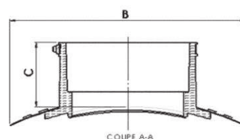
COUPE A-A
