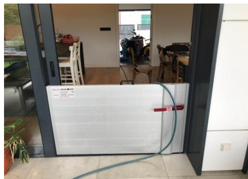
RAPID CLICK Entrada corredera largo 3,98, x 1m de alto y entrada valla peatonal de 1 m x 1m
